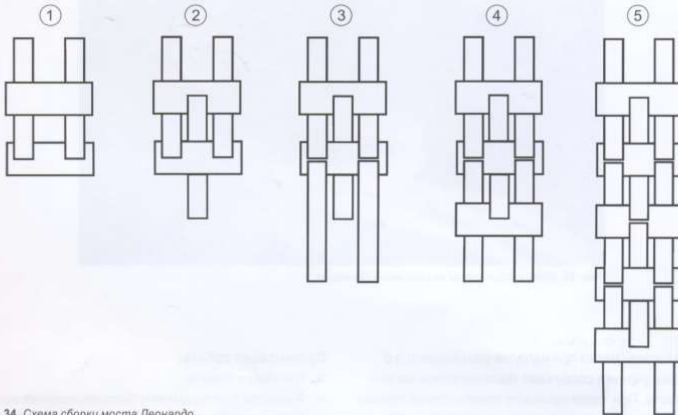
Рис. 34. Схема сборки моста Леонардо
